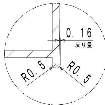
B拡大図 (3 : 1)
